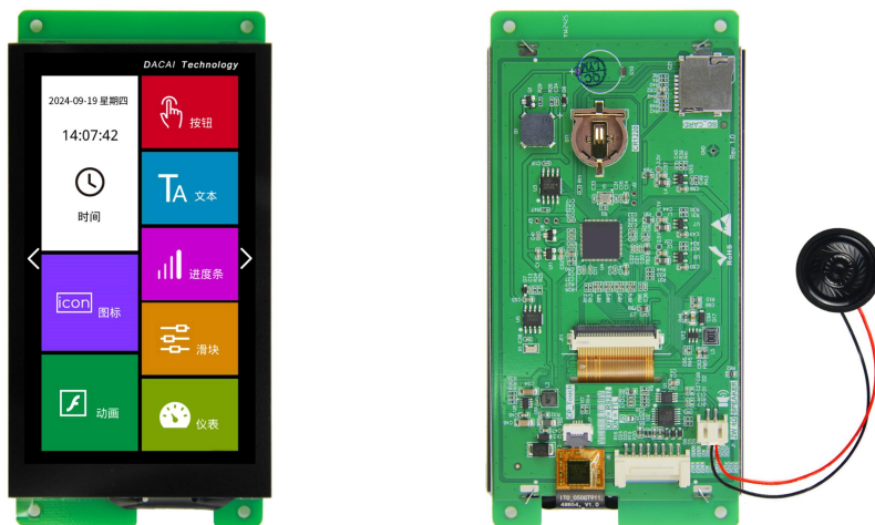
图 1-1 5.0 寸电容触摸参考图
