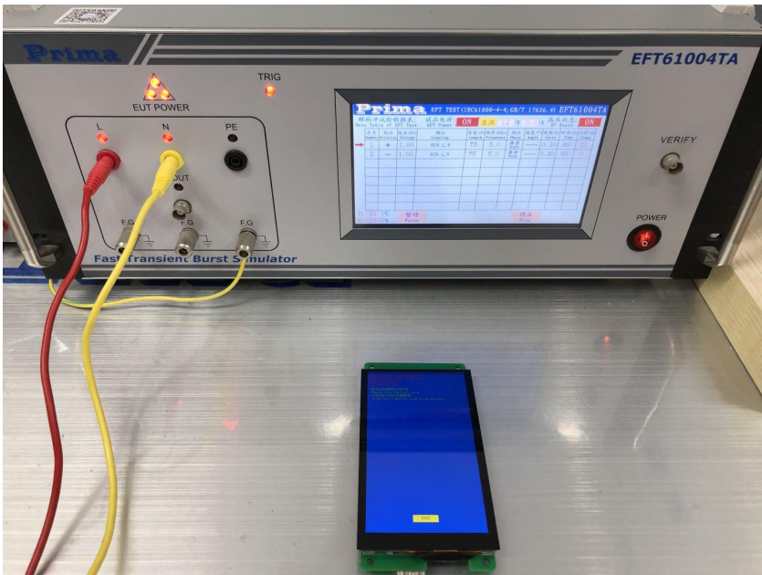
图 5-4 群脉冲测试图
