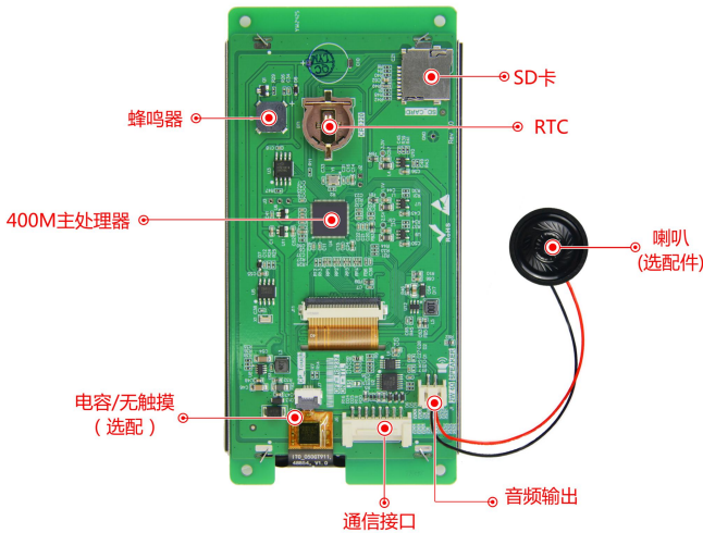
图 1-3 硬件配置图
